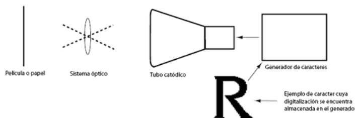
Figura 95.- Esquema de la fotocomponedora de la tercera generación.
