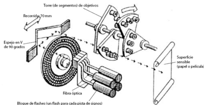
Figura 94.- Esquema de la fotocomponedora de la segunda generación.
